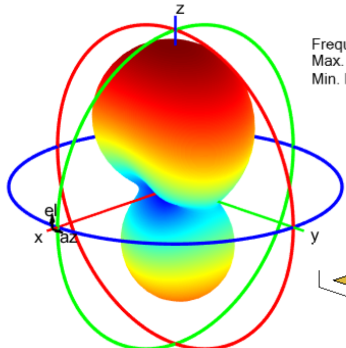
patchMicrostripEno tch
