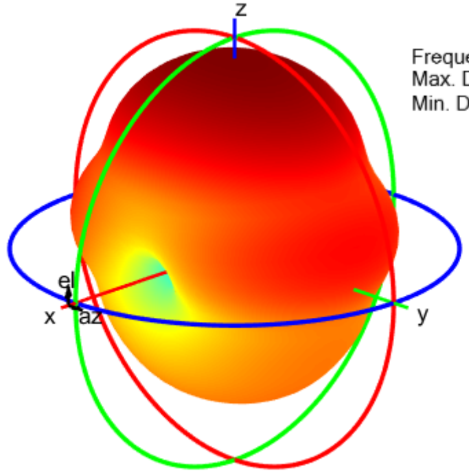
pifa
