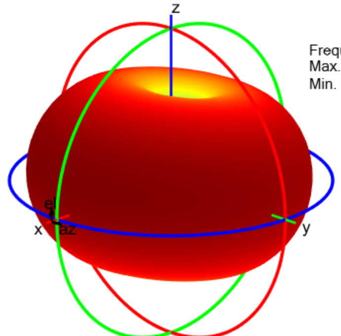
dipoleHelixMultifilar
